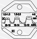
Installed Die
